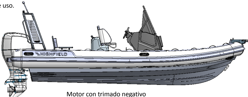
Motor con trimado negativo
