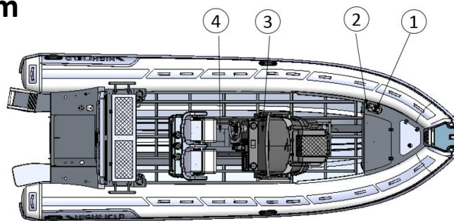
Darstellung Kraftstoffsystem
