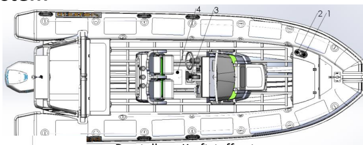
Darstellung Kraftstoffsystem
