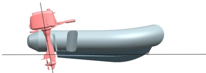
Bug nach unten, zu viel negative Trimmung
