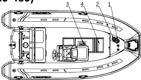
Darstellung Kraftstoffsystem
